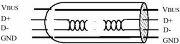
图 4.3-1 USB 电缆
